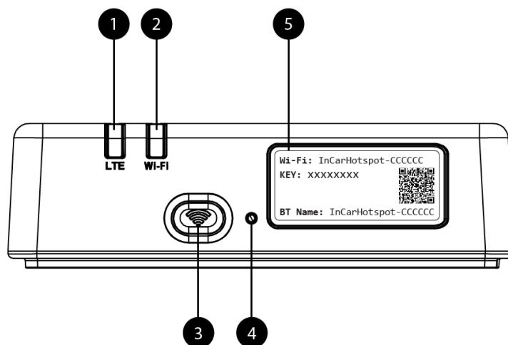
Рис. 1. Точка доступа Toyota Connected Services. Передняя панель
